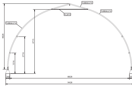
Päätykuvanto
